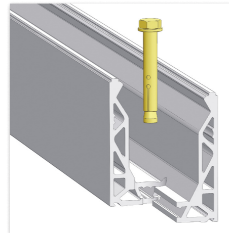
Entraxe des ancrages 200 mm
