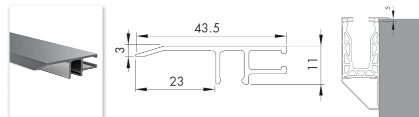
Garde-corps FenderStadium® en montage nez de dalle
